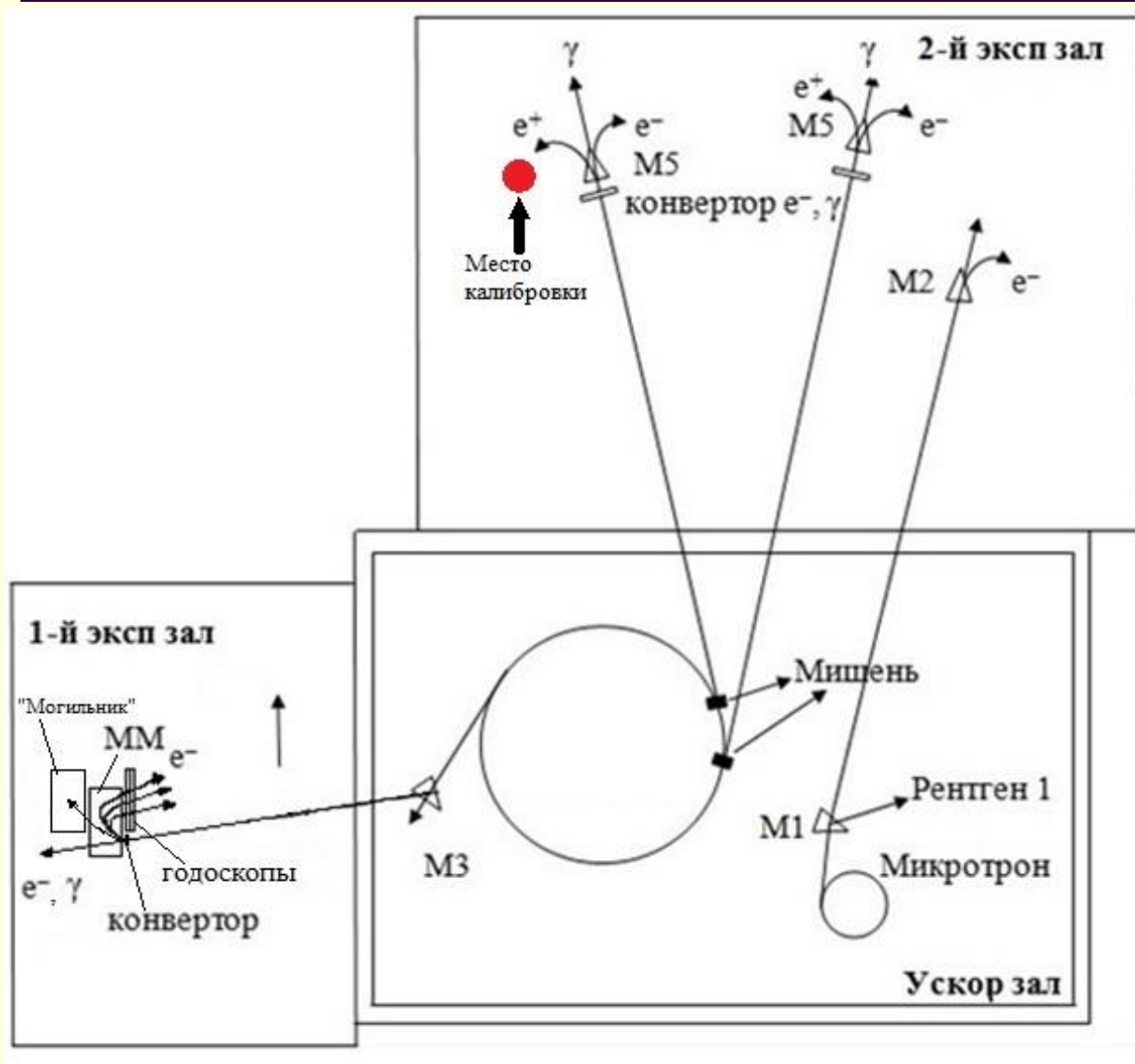
Рис. 2 Схема пучков ускорителя «Пахра»
