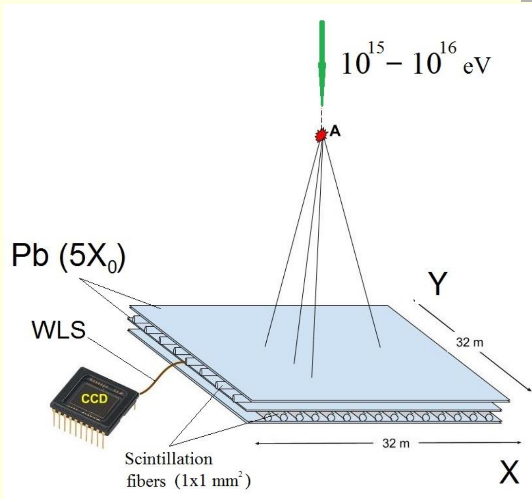
Рис. 1 Схема астротелескопа
